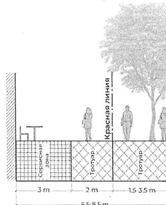
Пешеходный модуль тип 2
