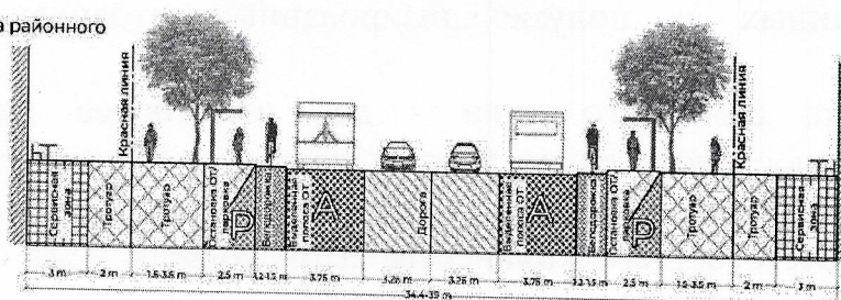
Магистральная улица районного значения тип 2
