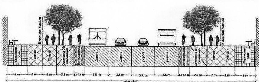
Магистральная улица районного значения тип 3
