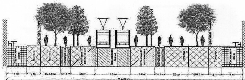
Бульвар с трамвайной линией тип 2
