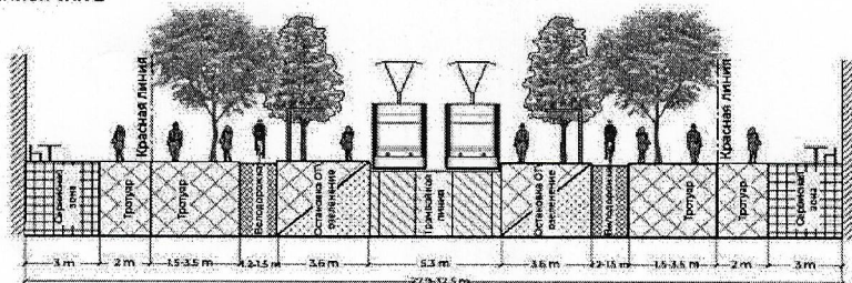
Бульвар с трамвайной линией тип 2
