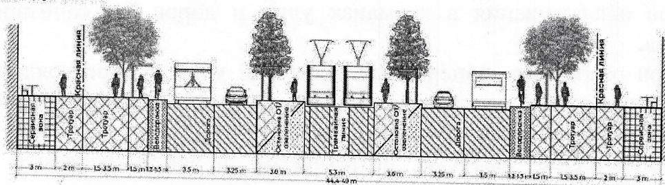
Магистральная улица тип 3
