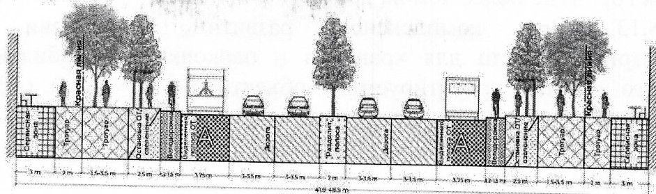
Магистральная улица тип 2
