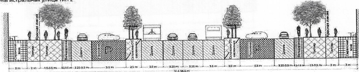
Магистральная улица тип 2
