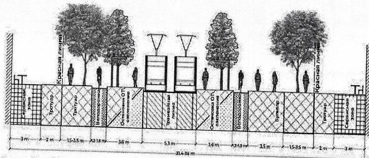
Бульвар с трамвайной линией тип 2
