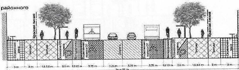
Магистральная улица районного значения тип 2
