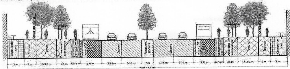
Магистральная улица тип 1
