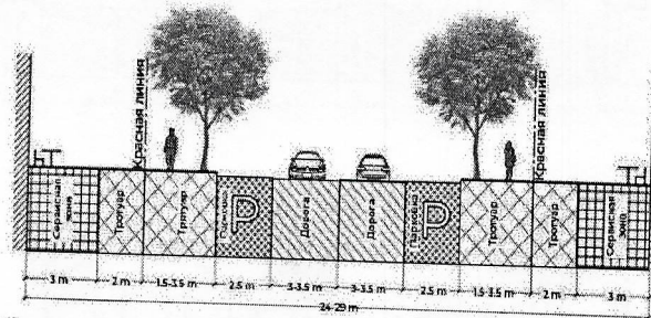
Улицы и дороги местного назначения тип 1
