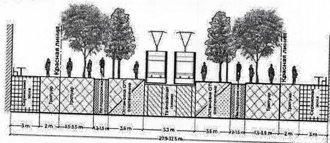
Бульвар с трамвайной линией тип 2
