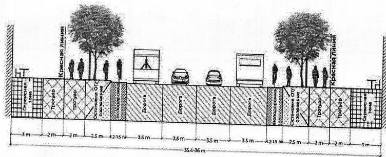
Магистральная улица районного значения тип 3
